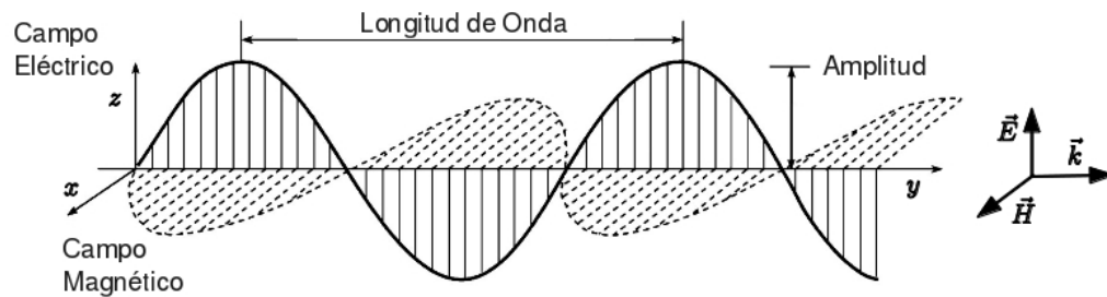
Figura 2.1: Onda 1D
